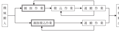
図 II ②-9 施工フロー
